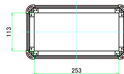
C-C ( 1 : 5.5 )
